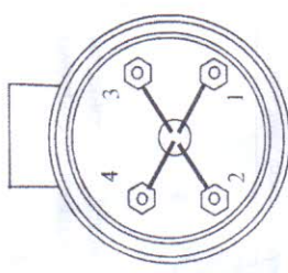
Рисунок 3. Нумерация клемм контактной колодки термообразователя.
